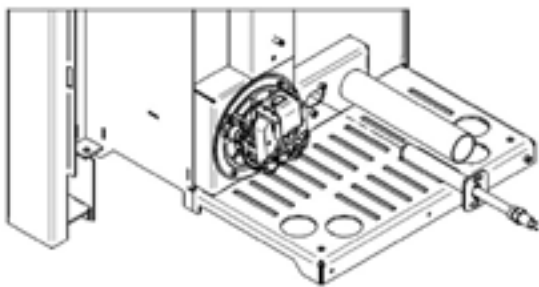
Afbeelding 3 - Ontsteker verwijderen
