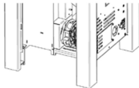
Afbeelding 4 - Ventilator verwijderen
