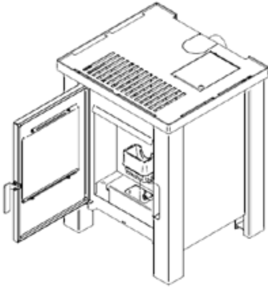
Figuur 1 - Brandpot
