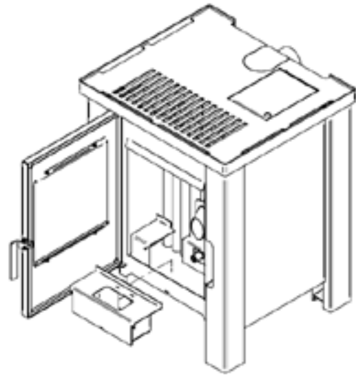
Figuur 2 - Brandpothouder
