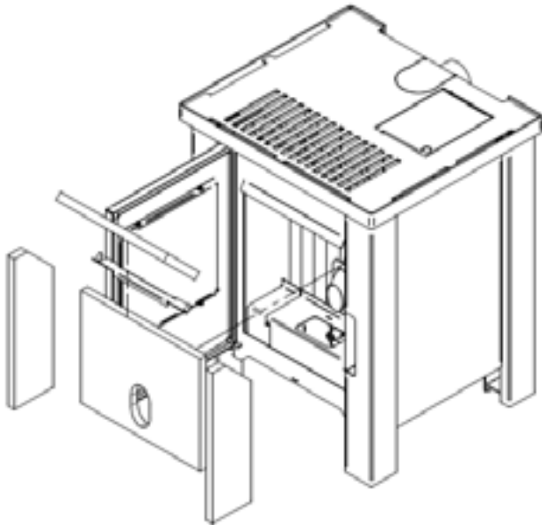
Figuur 3- Vermiculiet brandkamer
